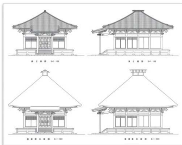
文化庁事業にて作成した大日堂現況図・復原図
